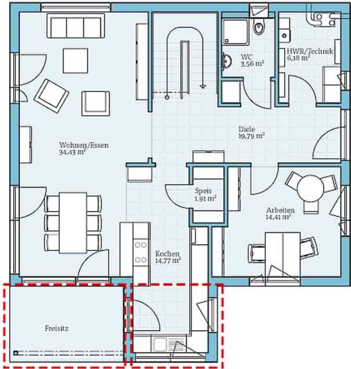
Grundriss Villa 177, Effizienzhaus 40+: EG
