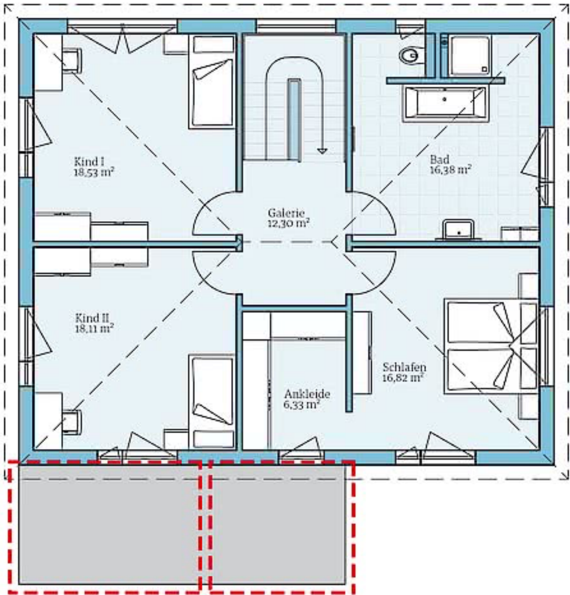
Grundriss Villa 177, Effizienzhaus 40+: OG
